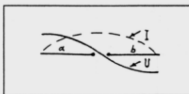
Abb. 1: Strom- und Spannungsverteilung in einer Dipol-Antenne.
