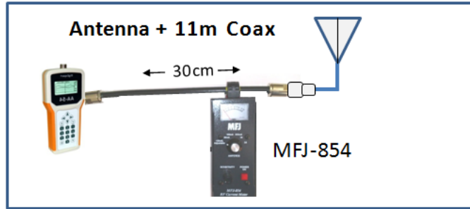
ANT TEST 1 Config. 1A
