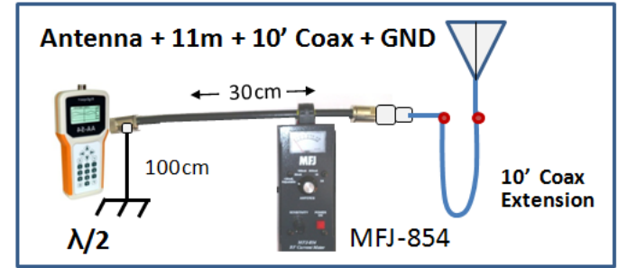
ANT TEST 6 Config. 2B
