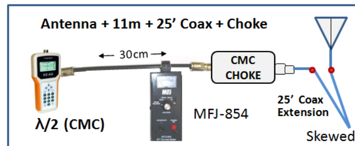
ANT TEST 15 Config. 4C
