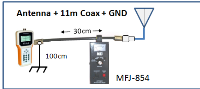
ANT TEST 2 Config. 1B
