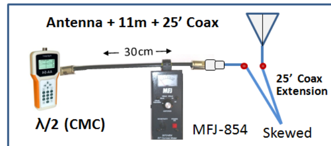
ANT TEST 13 Config. 4A
