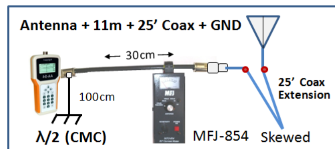
ANT TEST 14 Config. 4B
