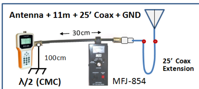
ANT TEST 10 Config. 3B
