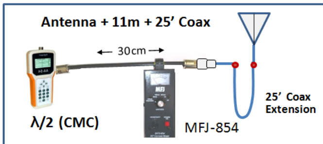
ANT TEST 9 Config. 3A
